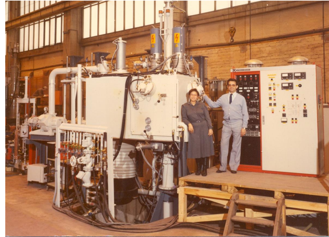
Forno piloto ES 2/18/300 CF, 18.000 L/s, 40 t/ano nominal
