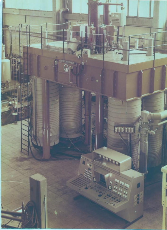
Forno de Fusão por Feixe de Elétrons ESP 300/1200 para lingotes de Nb e Ta, \varnothing = 400 mm; L = 2.000 mm; 300.000 L/min, 250 t/ano nominal
